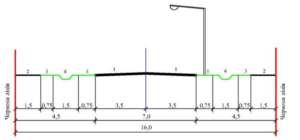
Житлові вулиці Розріз 2-2
