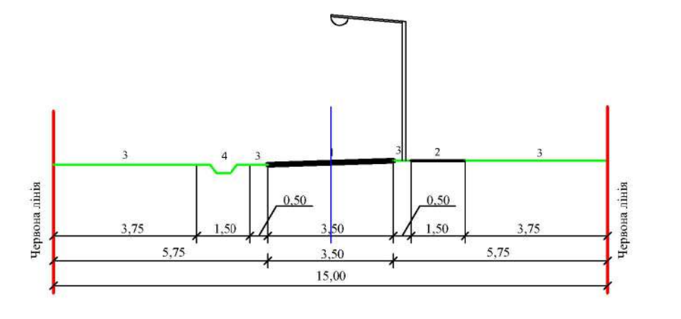
Житлові вулиці (Проїзди) Розріз 3-3
